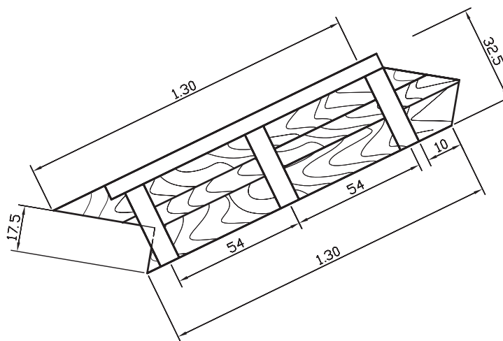
شکل ۶-۶- صفحه‌ی قالب گونده‌ی رامپ پله ۲ عدد
