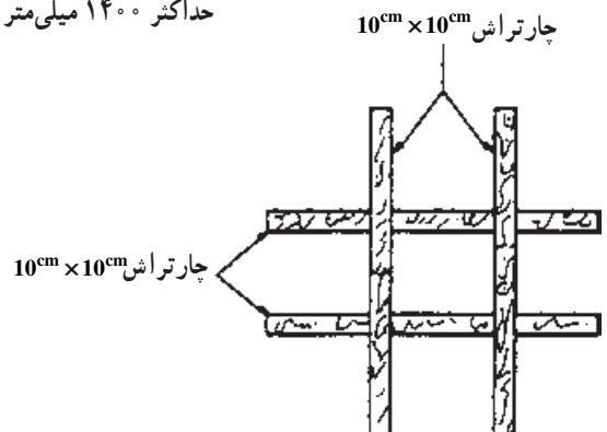
حدود ابعاد گیره - حداقل ۳۰۰ - حداکثر ۱۴۰۰ میلی متر
