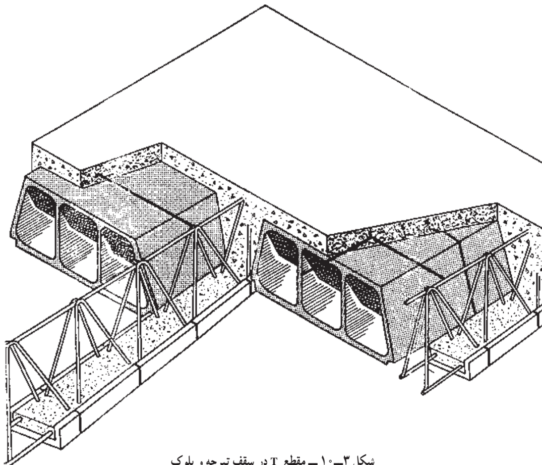
شکل ۳-۱۰ - مقطع T در سقف تیرچه و بلوک
