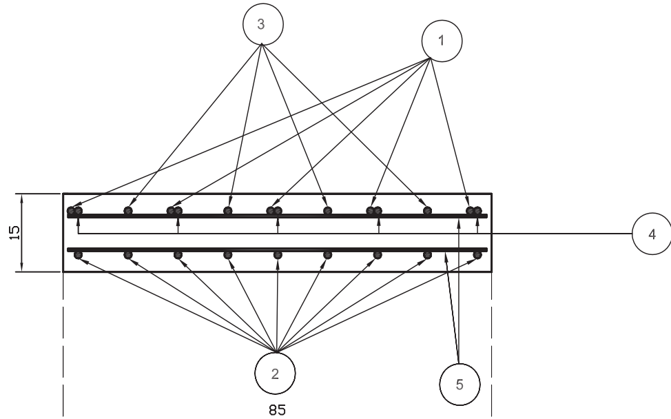
شکل ۱۵-۶- برش A-A
