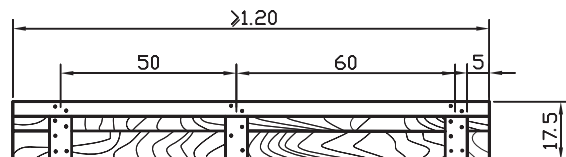
شکل ۸-۶- صفحه‌ی قالب گونده‌ی پاگرد پایین ۲ عدد
