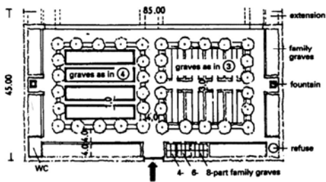
(۷) گورستان‌های مخصوص دهکده‌های بزرگ‌تر، یا در زمین نزدیک یک کلیسا، یعنی بدون در نظر گرفتن یک معدن مخصوص گورستان (پیشنهاد H. Hartwig)
