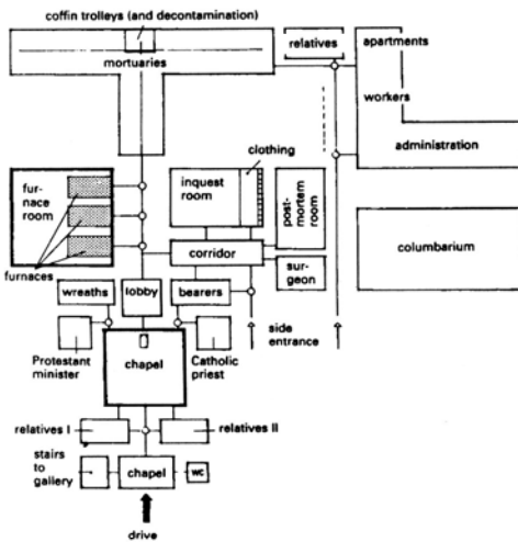
(۸) رابطه فضایی در یک گسالخانه با کوره سوزاندن اجساد و اتاق‌های جانبی برای یک گورستان بزرگ
