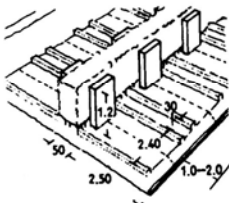
(۳) گورهای دویل، دیوارهای جدا کننده، راه رفت و آمد هم‌اکنون در سطح پایین‌تر
