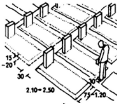
(۱) ترتیب گور سر به پا در قطعات با ۳۰۰-۳۰۰ گور
